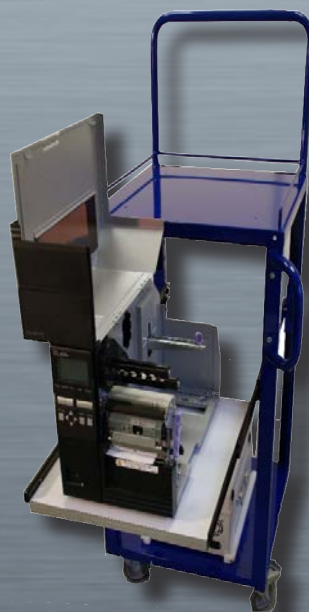
MOBIRACK avec tablette extractible avec loquet d'arrêt
