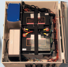
AGM Batterie
